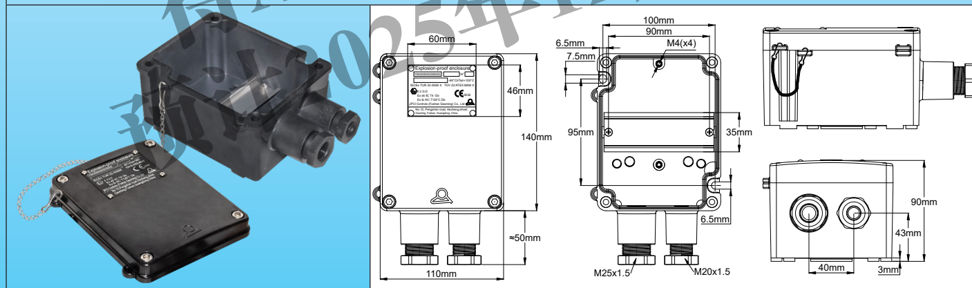
带导轨的示例
