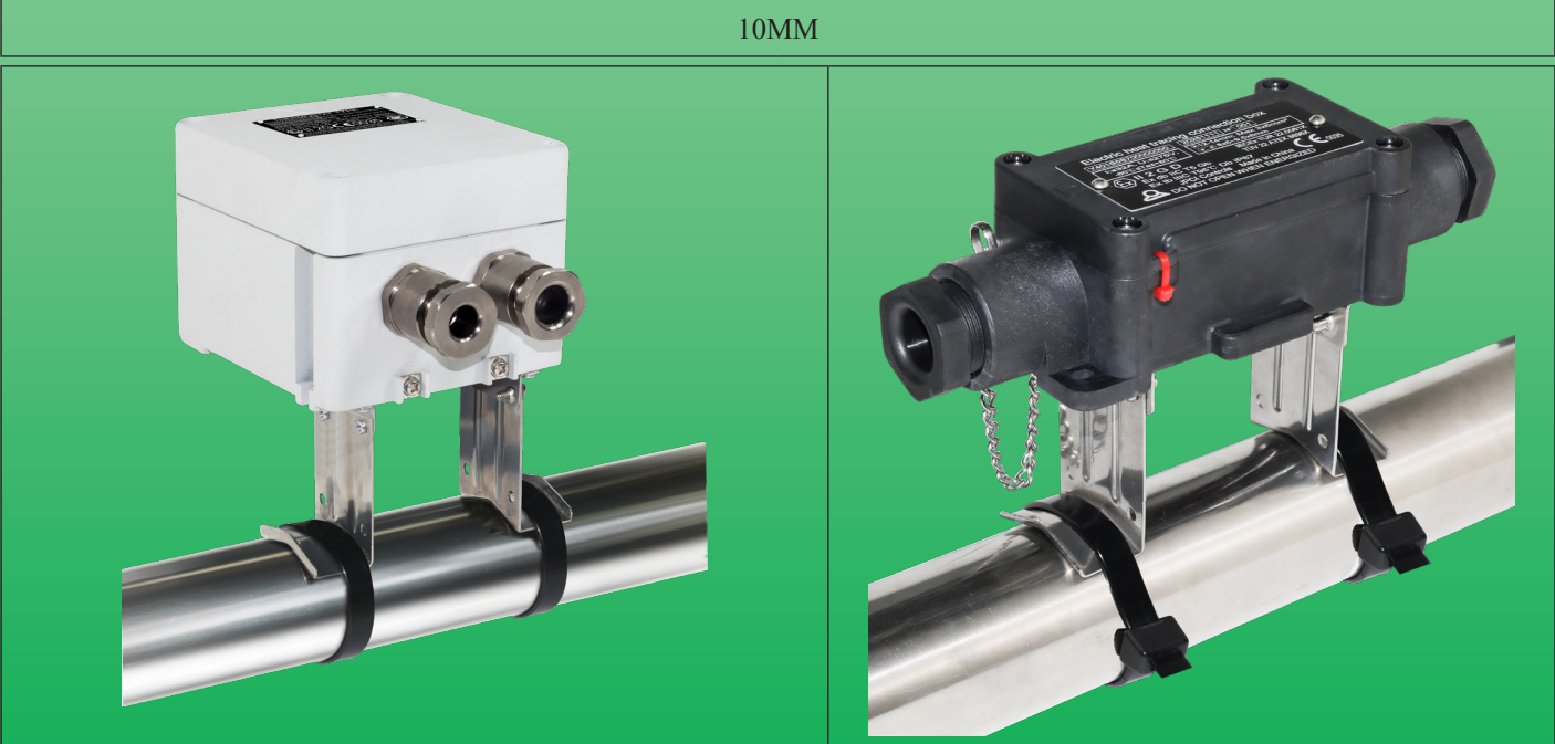
外壳140×110×90mm的组装示例 (型号 Y9)
